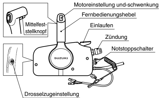
FERNBEDIENUNGSGEHÄUSE
